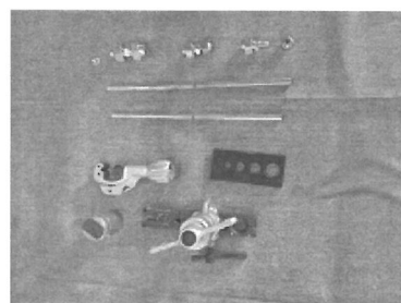
フレア加工
